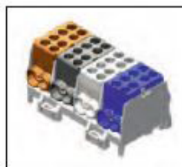
HLAK 35-4/8 BSG-S
